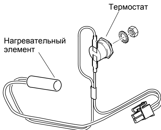
Система подогрева форсунки
