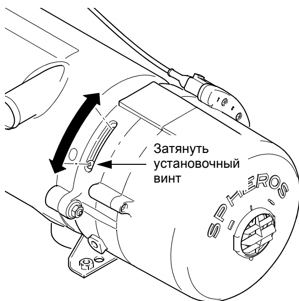
Рис. 702 Установочный винт для настройки содержания \text{CO}_2
