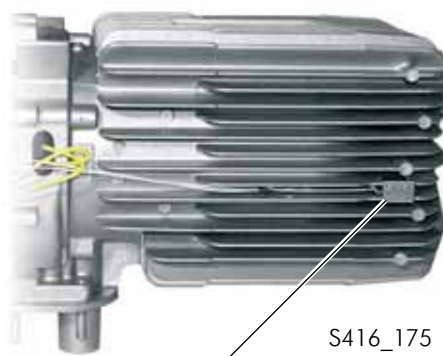
Датчик перегрева G189
