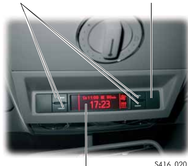
S416_020 Дисплей индикации дополнительного отопителя (на рисунке изображён Thermo Top C)
