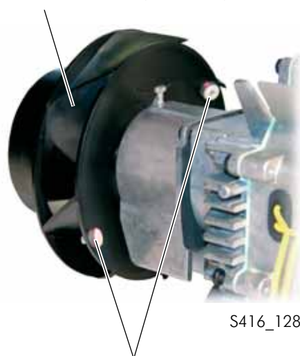
Постоянные магниты для определения частоты вращения вентилятора
