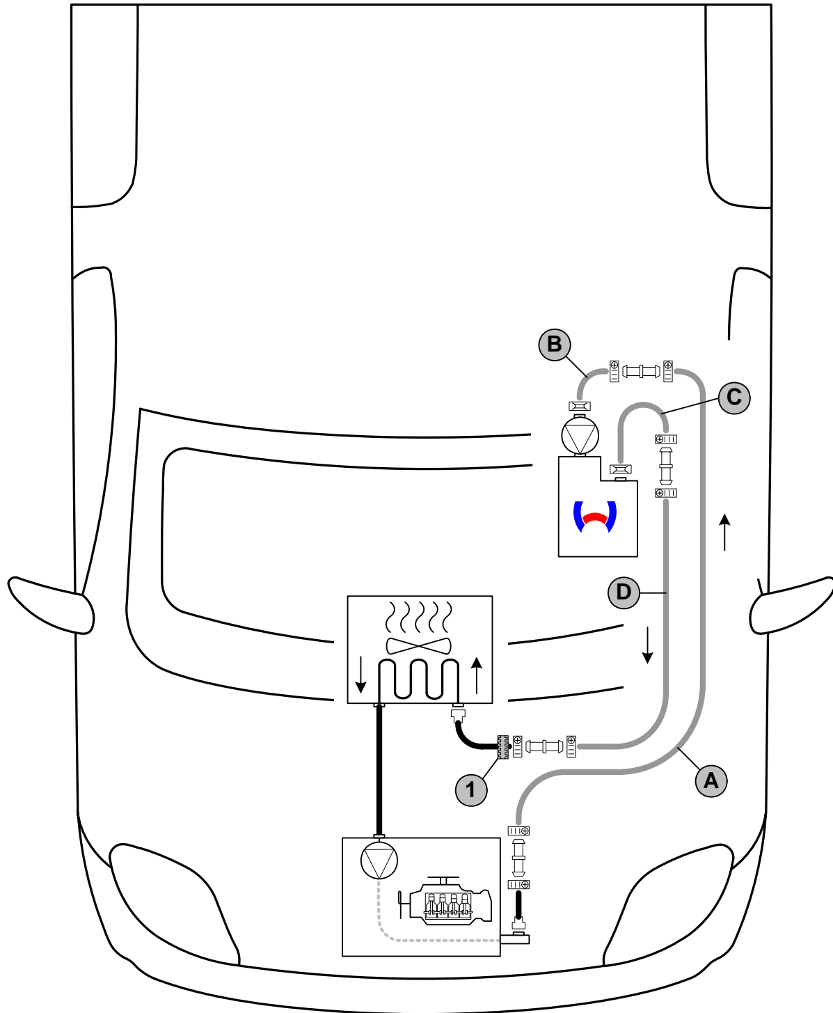
Schema Wasserverlegung
