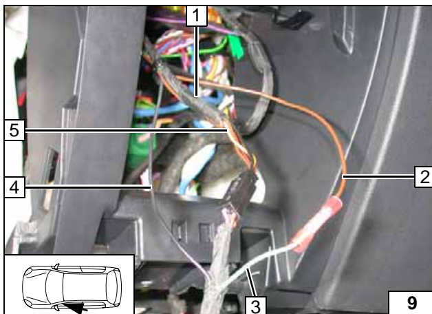
Abbildung zeigt Citroen C5! Verbindungen gemäß Schaltplan herstellen.
