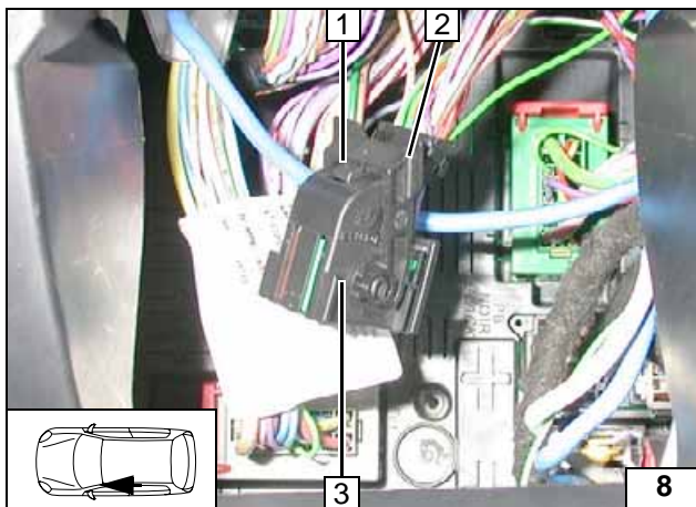
Abbildung zeigt Citroen C5! Verriegelung 1 eindrücken und Bügel 2 her- unterklappen.
