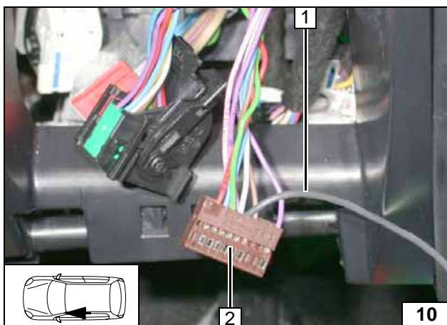
Abbildung zeigt Citroen C5! Anschluss am 20-poligen Stecker 2 vom BSI (Steckerfarbe kann variieren)! Microtimer von Ltg. sw 1 in PIN 6 einsetzen. Verbindungen gemäß Schaltplan herstellen.
