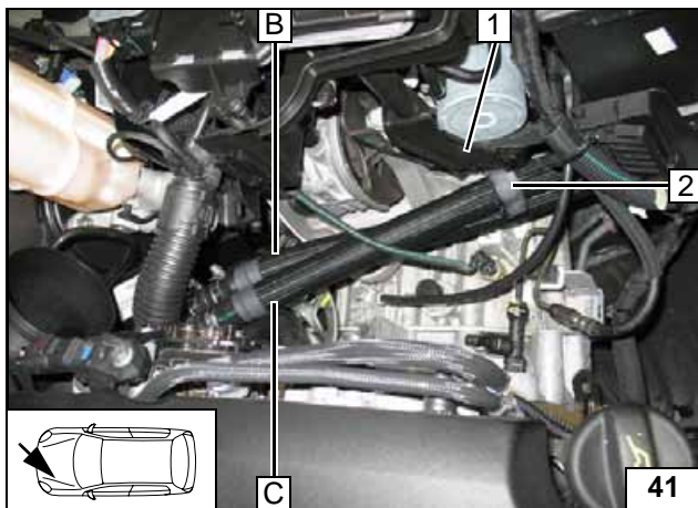
Profilgummi sw 2 mit Kabelbinder an Strebe 1 befestigen!
