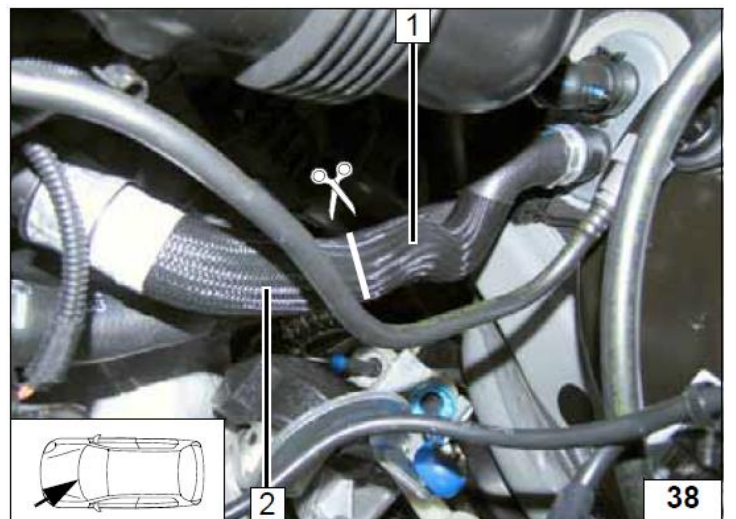
1 Часть патрубка на печку теплообменника 2 Часть патрубка с двигателя автомобиля
