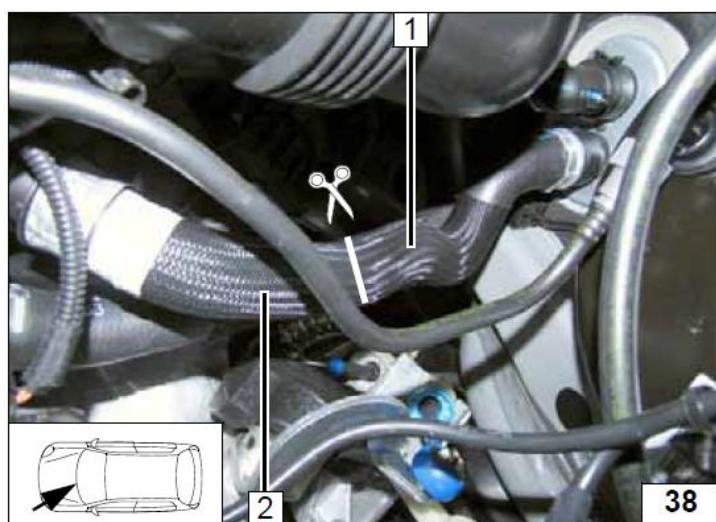
1 Часть патрубка на печку теплообменника 2 Часть патрубка с двигателя автомобиля
