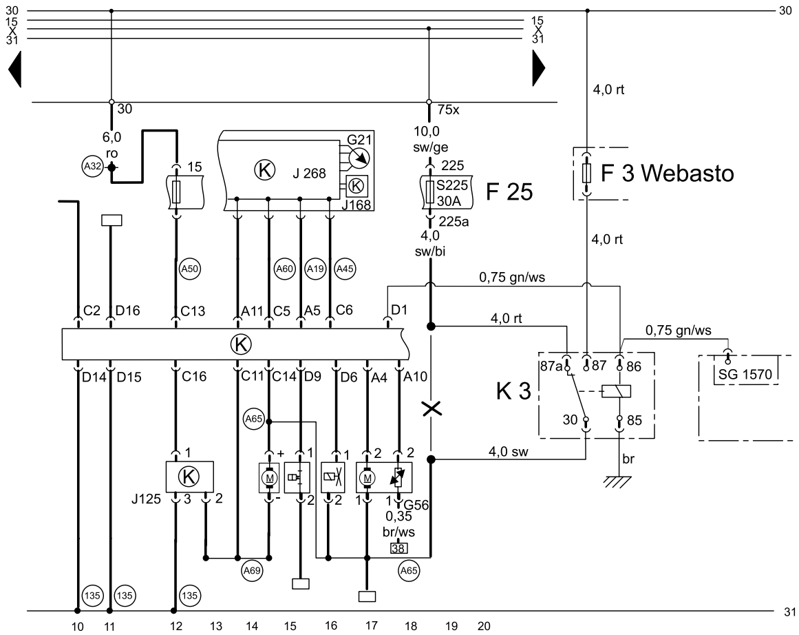
Schaltplan Gebläseansteuerung
