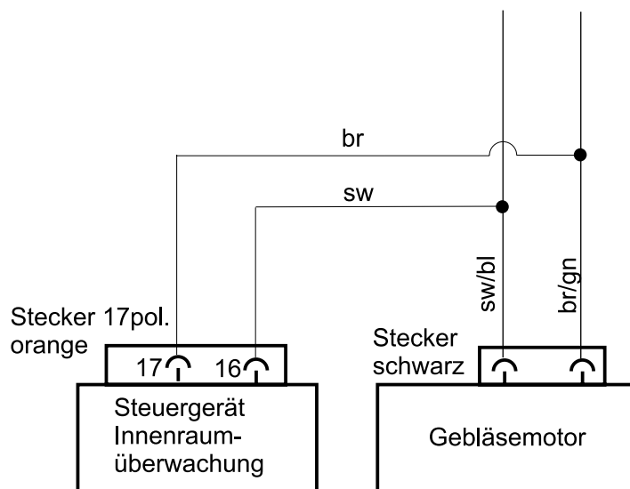
Schaltplan Innenraumüberwachung
