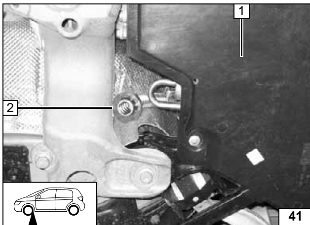
Unterfahrschutz 1 montieren.
